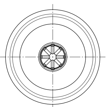
Ansicht Y
