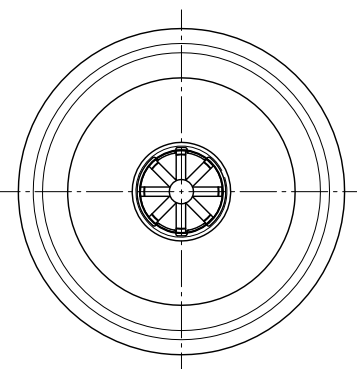
Ansicht Y
