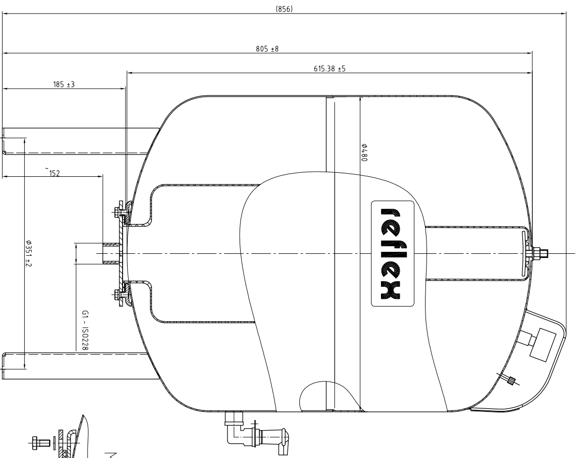
Montage Flansch
