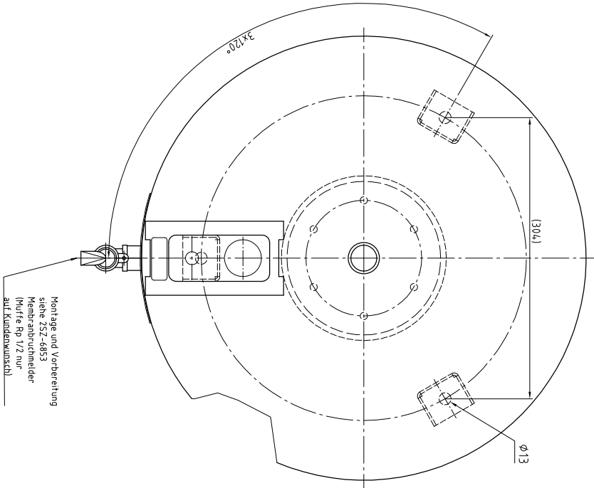
Montage Flansch
